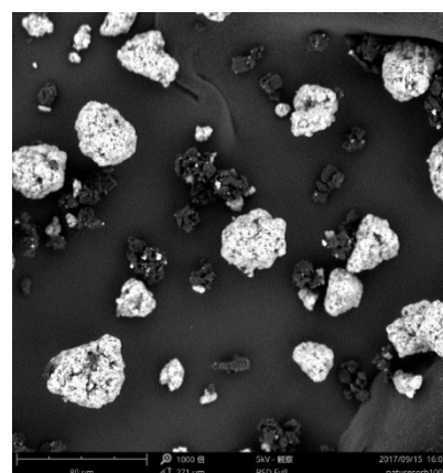
SEM 画像
