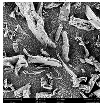
10μm 4900 倍
